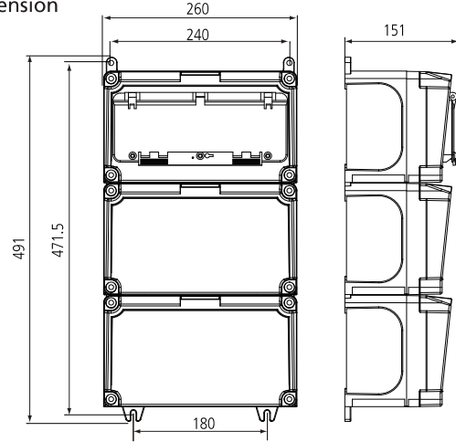
外形尺寸 Dimension
